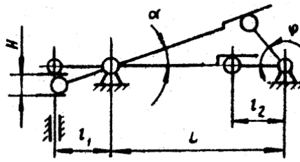
Рис. 17. Двухрычажный механизм с ведущей внутренней кулисой
