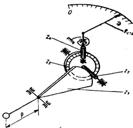
Рис. 16. Схема измерительной головки типа ИРБ
