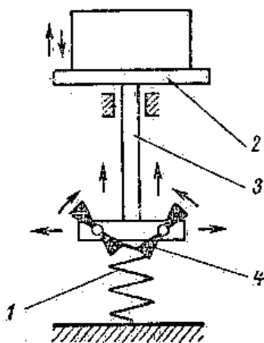
Рис.55. Принципиальная схема центробежного вибратора
