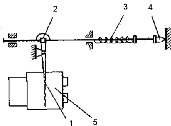
Рис.50. Схема ручного вибрографа
