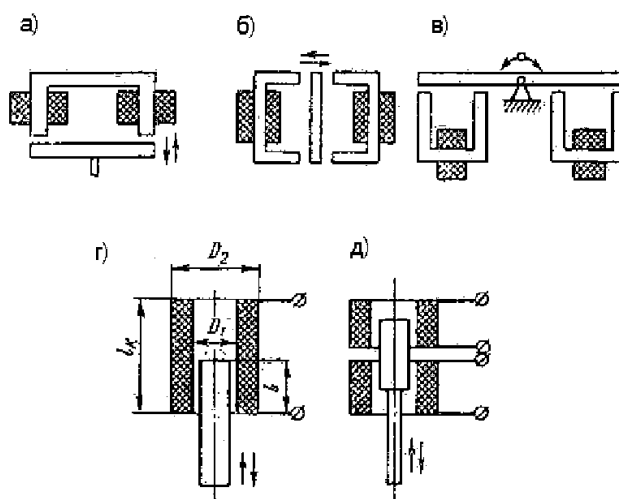
Рис. 46. Схематическое изображение индуктивных датчиков
