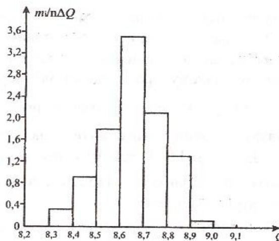
Рис. 32. Гистограмма, построенная по данным табл. 11
