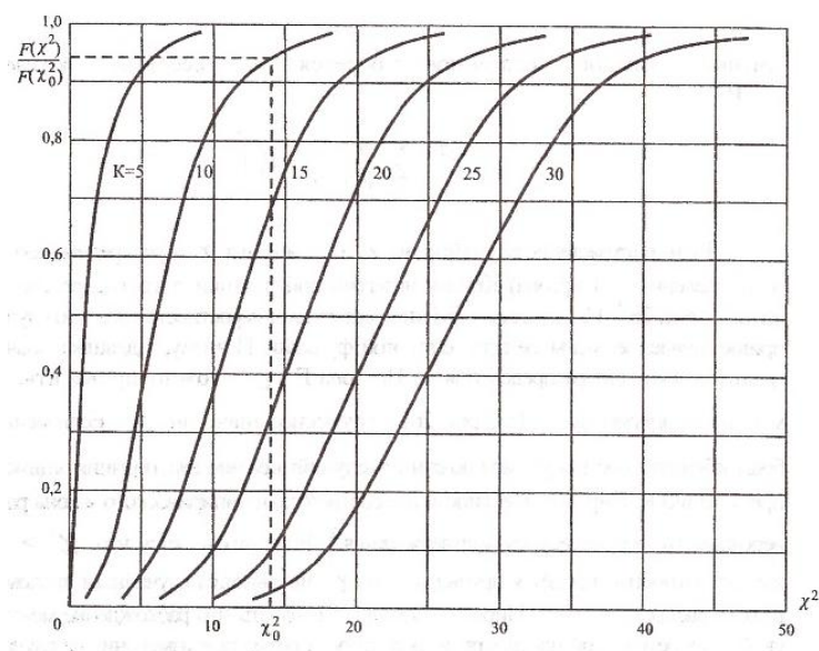
Рис. 31. Интегральная функция распределения вероятности К. Пирсона
