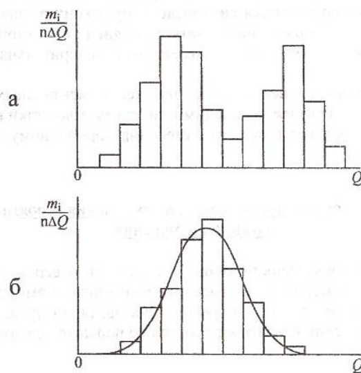
Рис. 30. Гистограммы, построенные по экспериментальным данным
