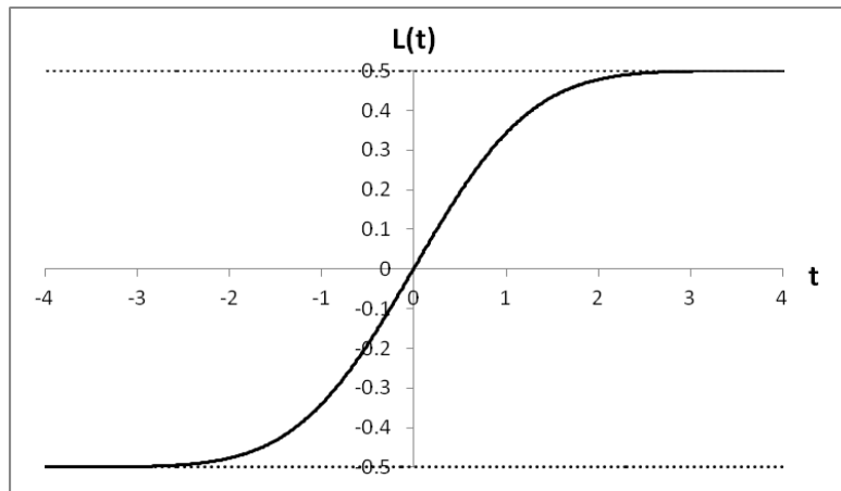
Рис.3. Функция Лапласа
