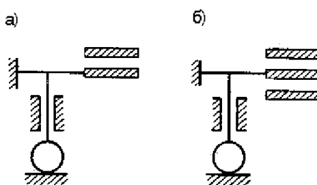
Рис.48. Принципиальные схемы простого(а) и дифференциального(б) емкостного датчика
