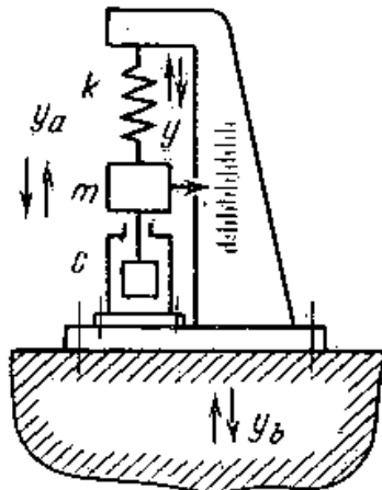
Рис. 37. Схематическое изображение чувствительного элемента
