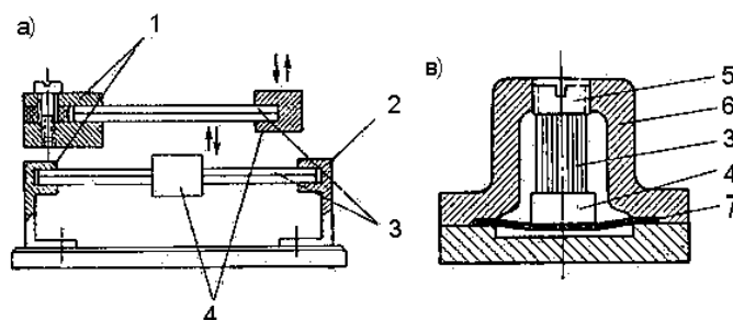
Рис. 44. Пьезопреобразователи: а — с биморфными пьезоэлементами, закрепленными консолью (вверху), и с двумя заделанными концами (внизу); б — с использованием поперечного пьезоэффекта
