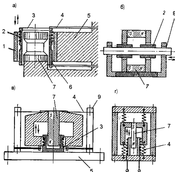
Рис. 42. Индукционные преобразователи
