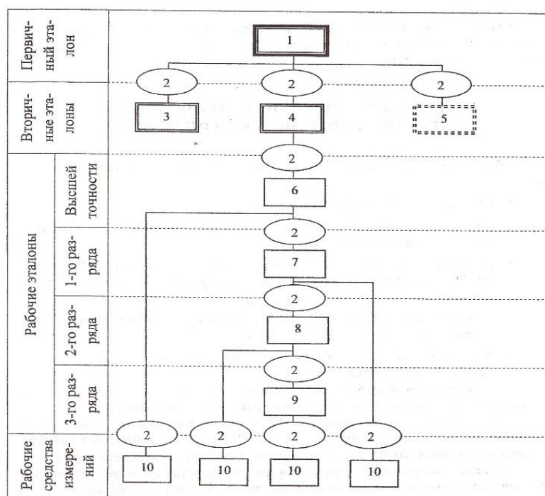
Рис. 35. Передача информации о размере единицы СИ (вариант): 1 - государственный первичный эталон; 2 - методы передачи информации о размере единицы; 3 - эталон сравнения; 4 - эталон-копия; 5 - эталон-свидетель; 6 - рабочий эталон высшей точности; 7, 8, 9 - рабочие эталоны соответствующих разрядов; 10 - средства измерений
