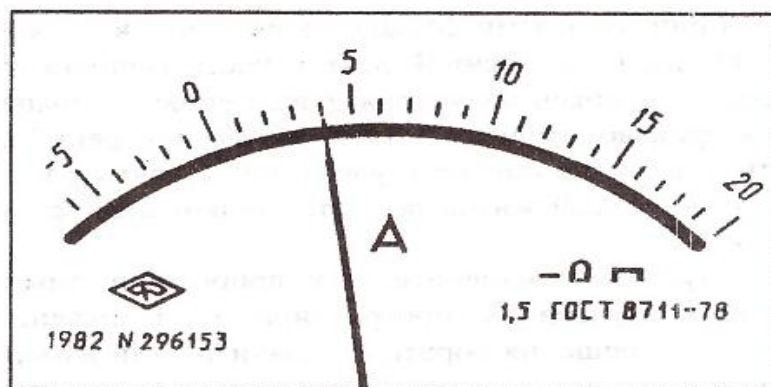
Рис. 22. Лицевая панель амперметра класса точности 1,5
