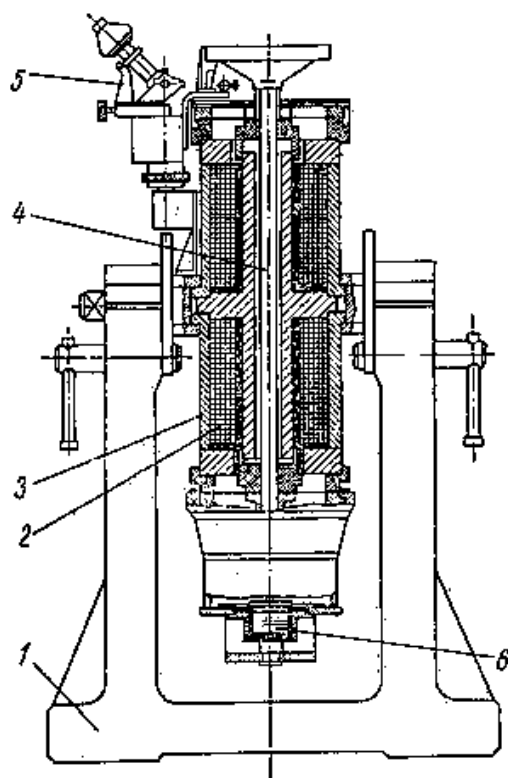
Рис. 58. Схема вибростенда типа ВС-300-П
