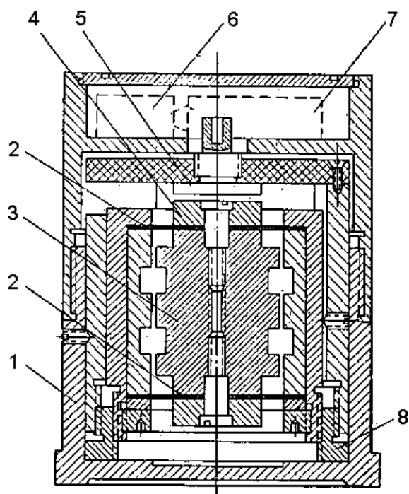
Рис. 51. Общий вид емкостного датчика
