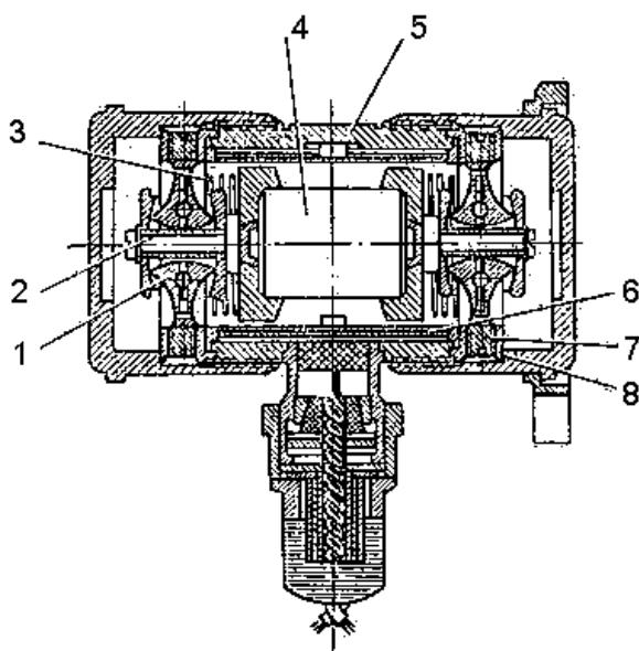
Рис.51. Общий вид индукционного датчика
