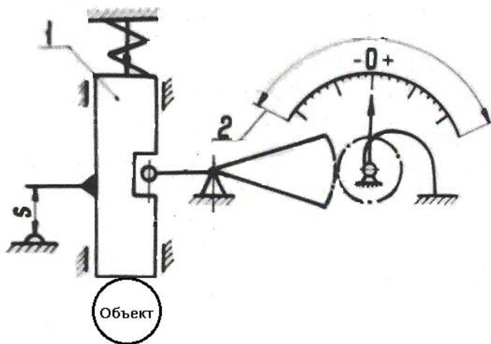
Рис. 8. Схема измерений
